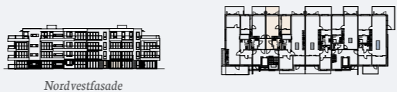
Nordvestfasade H04 - 103
